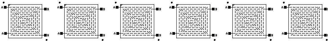
A-PBGA256-1.0MM-17MM-DC
